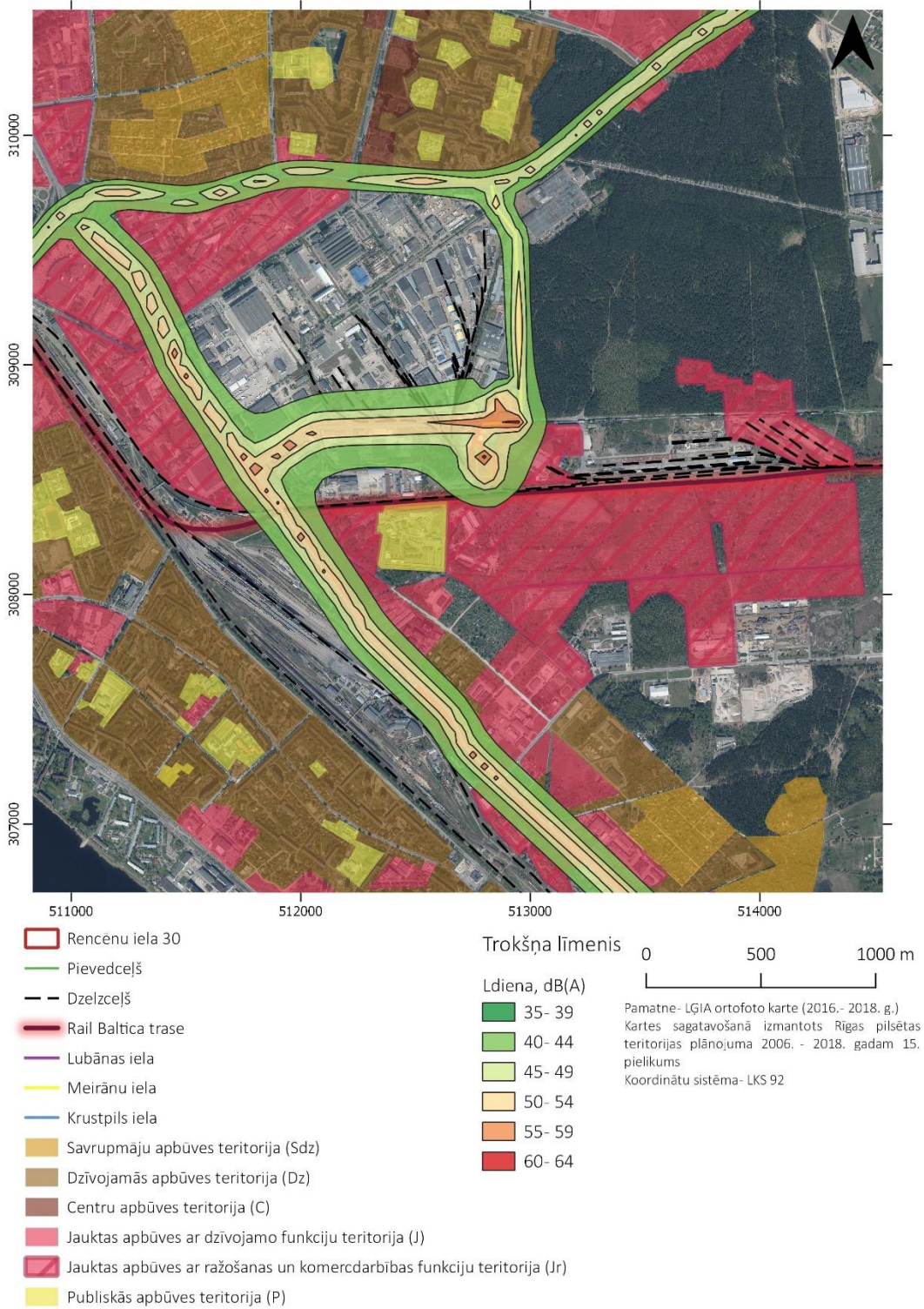
9.attēls. Operatora aprēķinātais trokšņa līmenis trokšņa rādītājam L_{diena}
